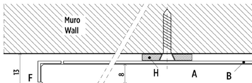
Sezione Orizzontale Horizontal section
