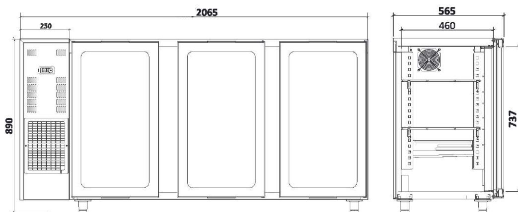
FGB 351/206 Imballo (mm)
